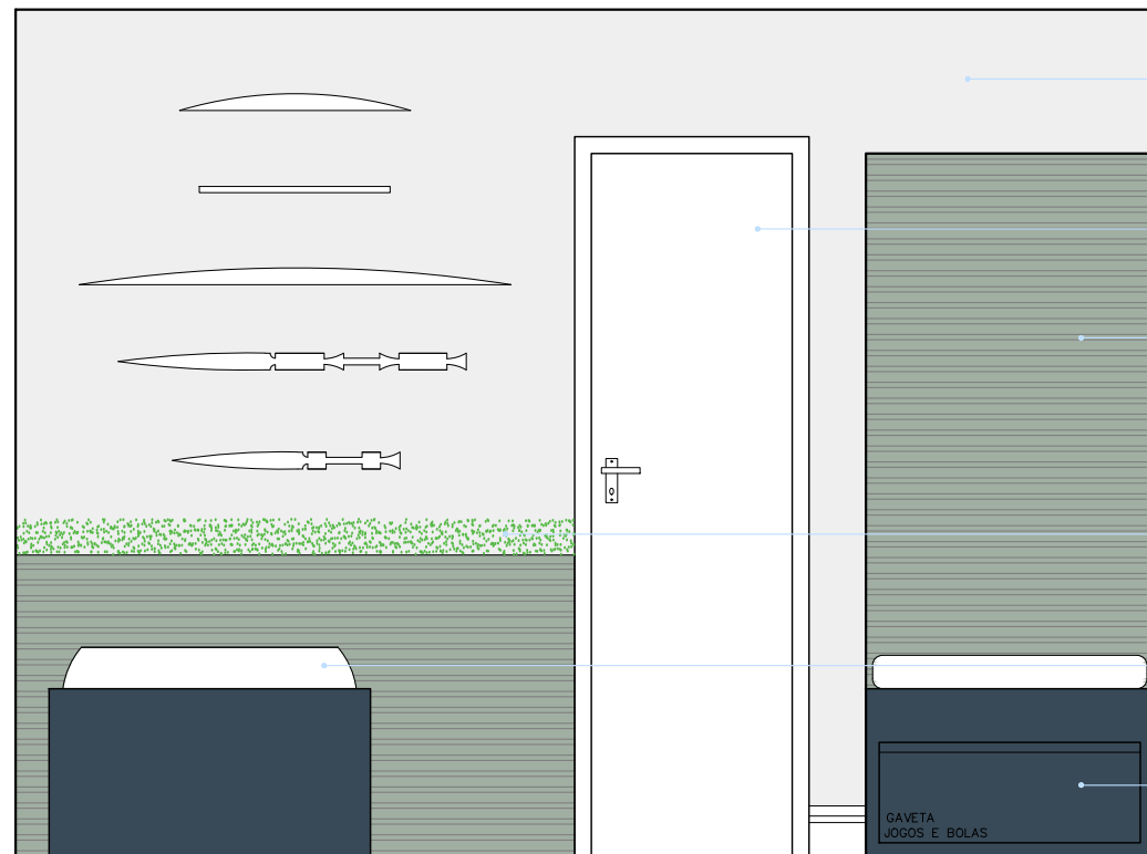
ELEVAÇÃO 03 ESC.1:25
