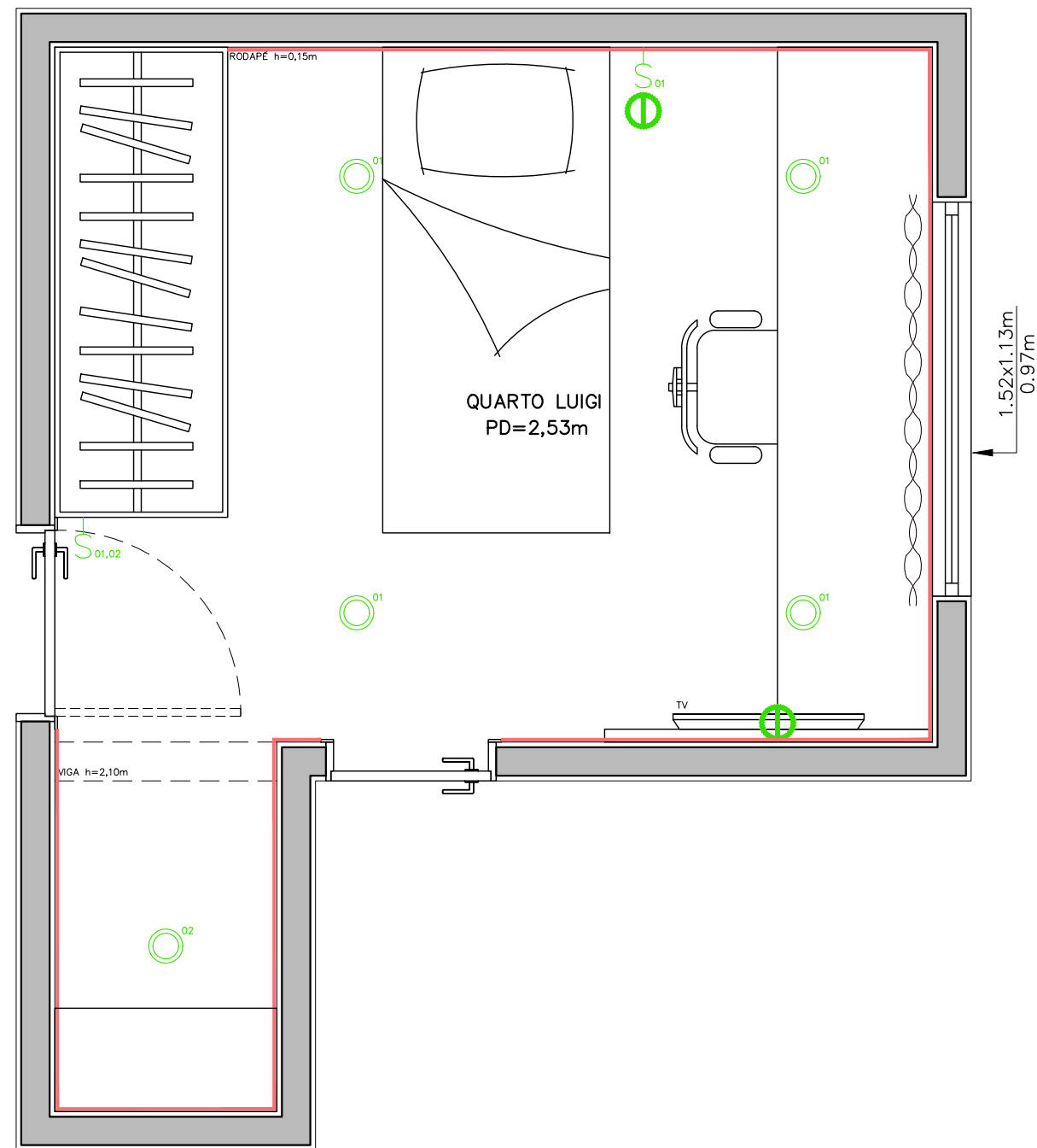
PLANTA DE LEVANTAMENTO ESC.1:25
